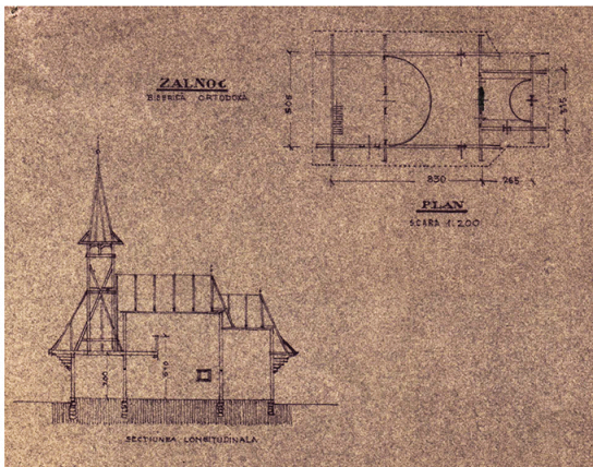
Biserica de lemn din Zalnoc, plan și secțiune (1963). Sursa: Culturalia.ro / Institutul Național al Patrimoniului
