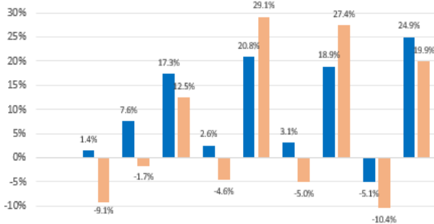
Istoric performanța
